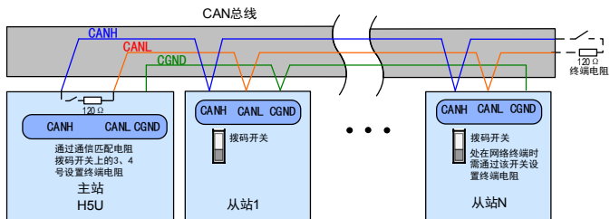
图 8 CANopen/CANlink 通讯连接示意图
