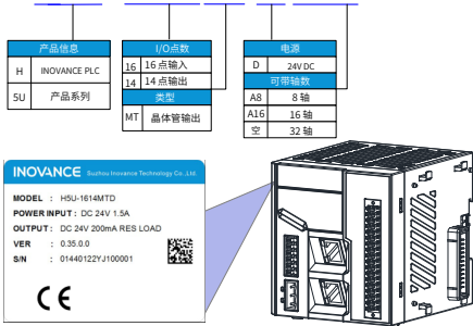
图 1 型号与铭牌说明
