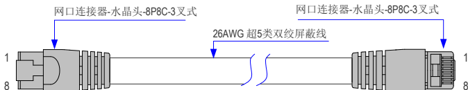
图 7 EtherCAT 网线制作要求
