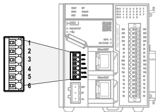
图 5 PLC 上的通讯端口定义
